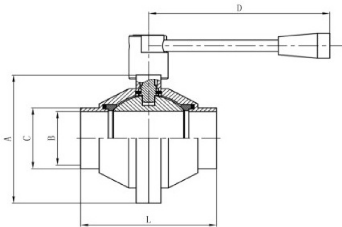
焊接式
