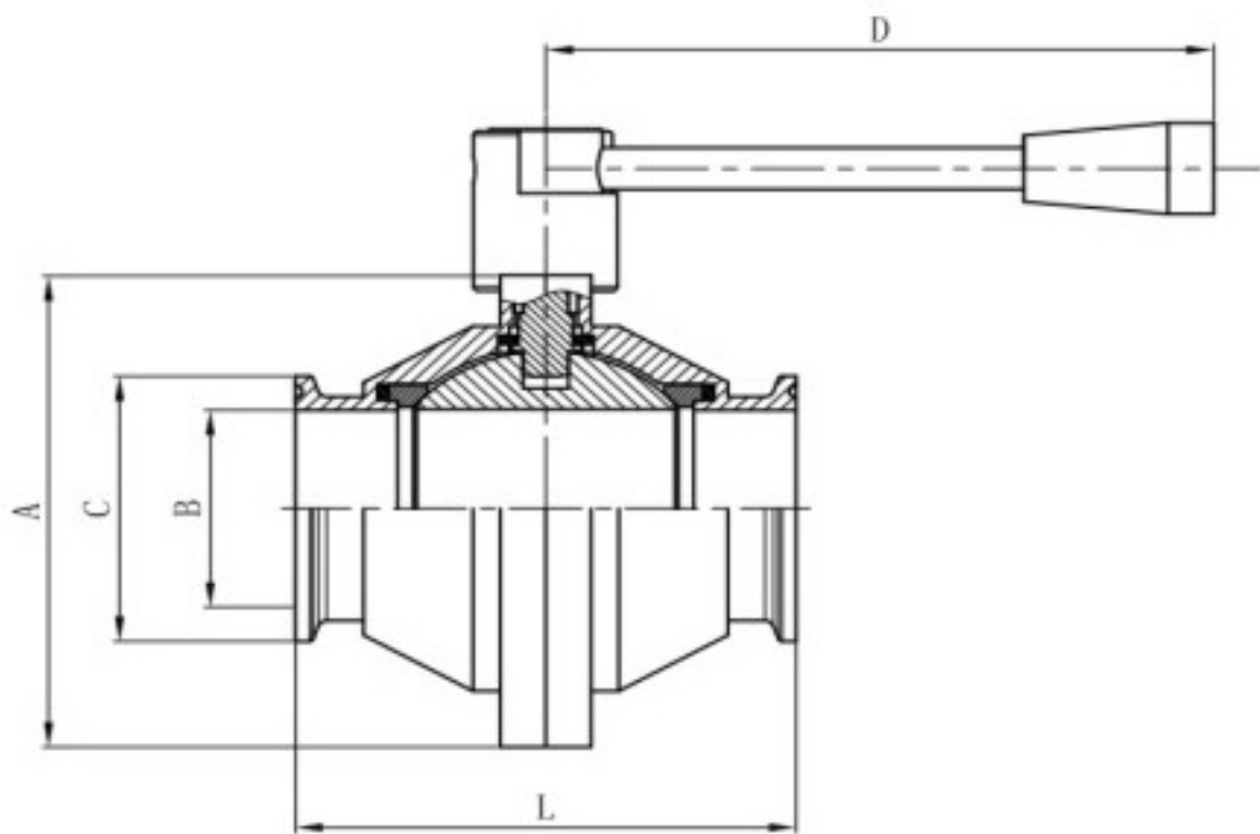
快装式
